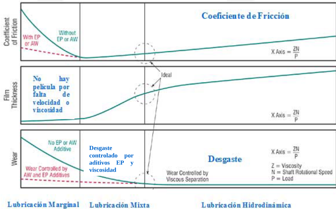
Fig. 9 Coeficiente de fricción, espesor de película de aceite y desgaste según el tipo de lubricación
