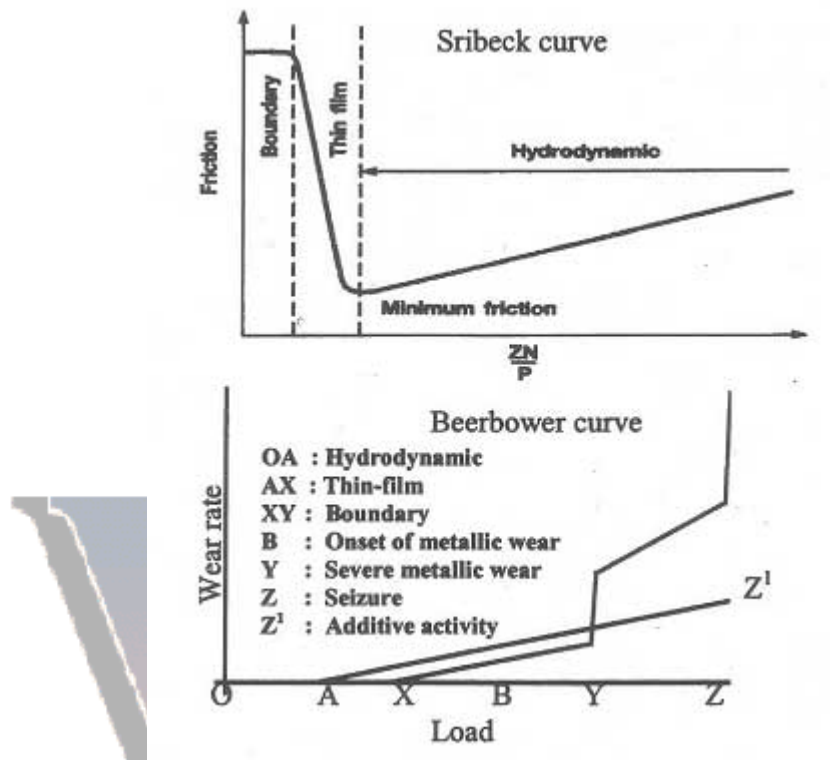
Fig. 9 Stribeck y Beerbower
