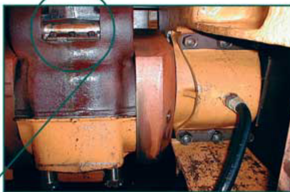
Figura 3. Biela y contrapesos
